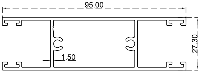
قاطع اباور (27.3*95) ملم الرقم التسلسلي للصنف: BLT886 الوزن 1.168:(Kg/m)
