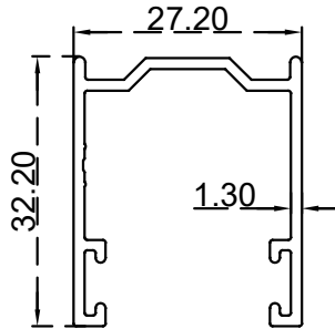
يو مع فرشاية (32.2*27.2) ملم الرقم التسلسلي للصنف: AS00028 الوزن 0.375:(Kg/m)
