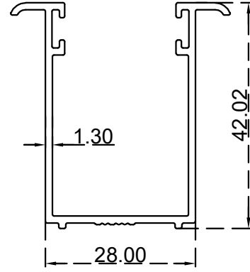
يو حلق صاج مكتساف (28*42.02) ملم الرقم التسلسلي للصنف: BLT3899 الوزن 0.483:(Kg/m)
