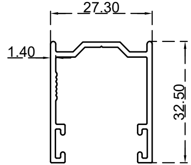
يو مع فرشاية (27.3*32.5) ملم الرقم التسلسلي للصنف: BLT391 الوزن 0.420:(Kg/m)
