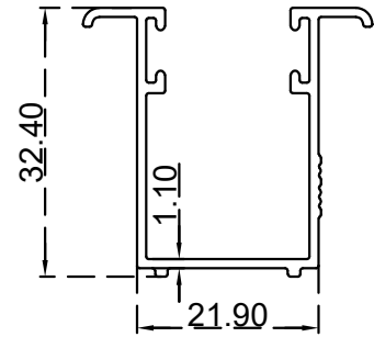
يو حلق صاج تريپس اور (21.9*32.4) ملم الرقم التسلسلي للصنف: BLT1648 الوزن 0.349:(Kg/m)
