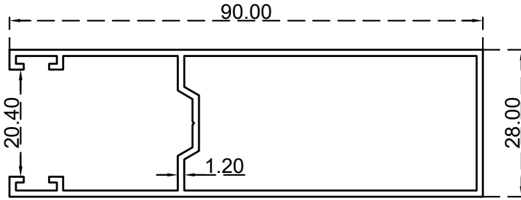
يو منوبلوك (28*90) ملم الرقم التسلسلي للصنف: BLT039 الوزن 0.817:(Kg/m)
