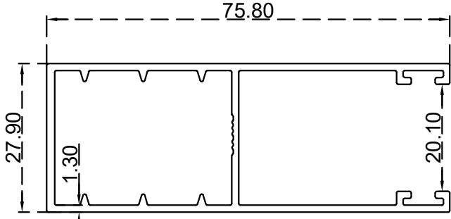
يو منوبلوك (27.9*75.8) ملم الرقم التسلسلي للصنف: BLT882 الوزن 0.817:(Kg/m)
