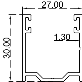
يو مع فرشاية (27*30) ملم الرقم التسلسلي للصنف: AS00010 الوزن 0.362:(Kg/m)
