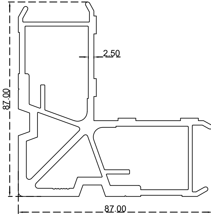
زاوية تجميع 36 ملم إكسنتال الرقم التسلسلي للصنف: BLT4654 الوزن 3.071:(Kg/m)
