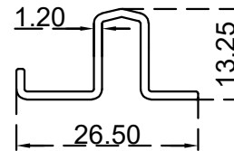
يو زجاج دبل الرقم التسلسلي للصنف: BLT495 الوزن: 0.166:(Kg/m)
