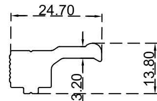
موصل زجاج عزل الطبقة الداخلية الرقم التسلسلي للصنف: BLT4331 الوزن: 0.457:(Kg/m)
