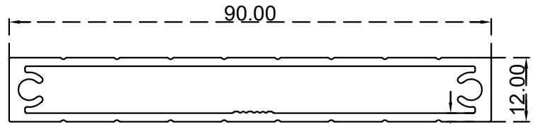
حلق مخفي 90 ملم الرقم التسلسلي للصنف: BLT4405 الوزن (Kg/m): 0.952
