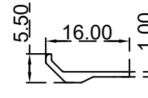
حامل زجاج الرقم التسلسلي للصنف: BLT496 الوزن: 0.254:(Kg/m)
