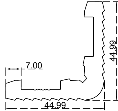
زاوية تجميع خاص 45 ملم الرقم التسلسلي للصنف: BLT4810 الوزن 1.434:(Kg/m)
