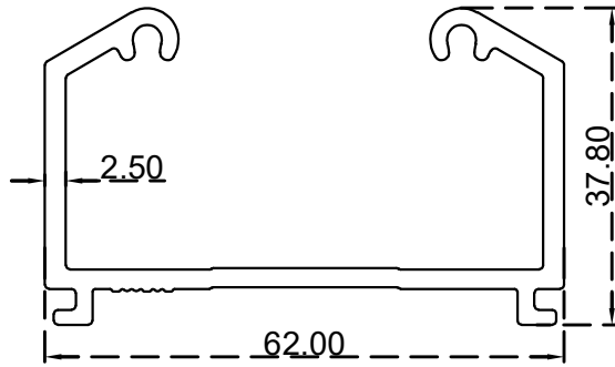
شبرتس قاطع 2000 خاص الرقم التسلسلي للصنف: BLT4864 الوزن (Kg/m): 1.047
