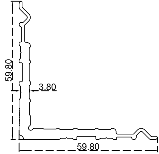
زاوية تجميع 4300-7300-7500 الرقم التسلسلي للصنف: BLT4632 الوزن 1.023:(Kg/m)
