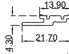
فلاخ سيكا الرقم التسلسلي للصنف: BLT1876 الوزن: 0.134:(Kg/m)
