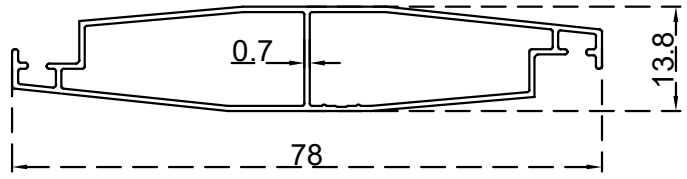
شلاف 80 ملم خفيف الرقم التسلسلي للصنف: AS00094 الوزن 0.360:(Kg/m)
