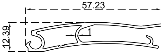
شلاف اور 57.23 ملم الرقم التسلسلي للصنف: BLT3278 الوزن 0.388:(Kg/m)
