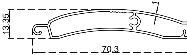
شلاف اور 70 ملم مع برغي الرقم التسلسلي للصنف: BLT5133 الوزن 0.450:(Kg/m)
