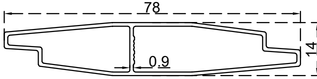
شلاف 80 ملم الرقم التسلسلي للصنف: BLT4784 الوزن 0.473:(Kg/m)
