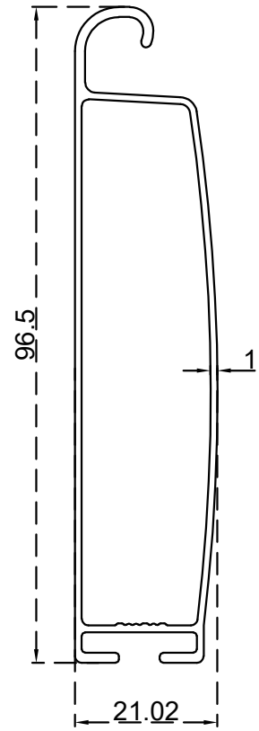
شلاف سوقييت 96.5 ملم الرقم التسلسلي للصنف: BLT4988 الوزن 0.688:(Kg/m)
