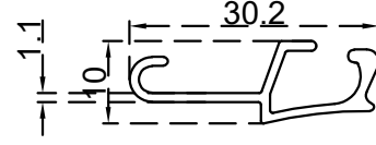
وصلة شلاف الرقم التسلسلي للصنف: BLT986 الوزن 0.179:(Kg/m)
