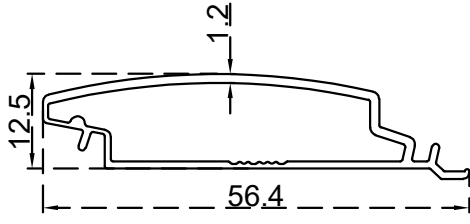
شلاف 50 ملم خاص الرقم التسلسلي للصنف: BLT4726 الوزن 0.344:(Kg/m)
