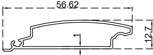
شلاف 50 ملم الرقم التسلسلي للصنف: ZD009B الوزن 0.328:(Kg/m)
