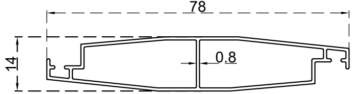
شلاف 80 ملم الرقم التسلسلي للصنف: BLT1805 الوزن 0.408:(Kg/m)
