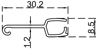
وصلة شلاف اور 55 ملم الرقم التسلسلي للصنف: BLT237 الوزن 0.153:(Kg/m)
