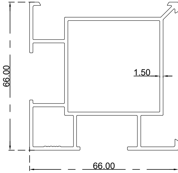
اطار باب زاوية مع غطاء الرقم التسلسلي للصنف: BLT3654 الوزن 1.364:(Kg/m)
