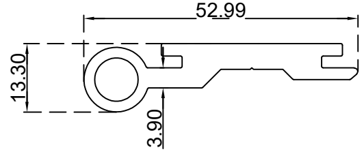
مفصلة باب الرقم التسلسلي للصنف: BLT1958 الوزن 0.809:(Kg/m)
