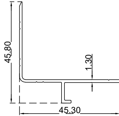
زاوية باب 45.8*45.29 ملم الرقم التسلسلي للصنف: BLT4624 الوزن 0.306:(Kg/m)
