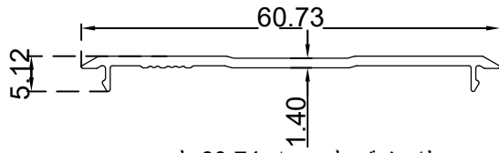
غطاء دفعة وحلق جدار 60.74 ملم الرقم التسلسلي للصنف: BLT4281 الوزن 0.246:(Kg/m)
