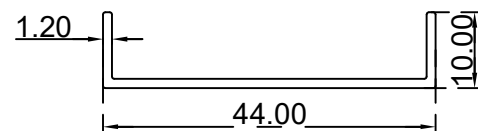
يو 1.2*10*44 ملم الرقم التسلسلي للصنف: C44X10X1.2 الوزن 0.200:(Kg/m)
