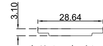
سبيسر دفعة و حلق جدار 40 ملم الرقم التسلسلي للصنف: BLT4286 الوزن 0.210:(Kg/m)
