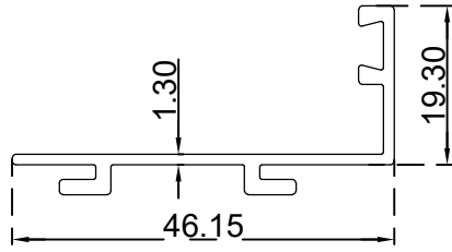
رداد باب 40 ملم الرقم التسلسلي للصنف: BLT4288 الوزن 0.341:(Kg/m)
