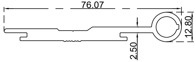
مفصلة دفة و حلق 59.67 ملم الرقم التسلسلي للصنف: BLT4618 الوزن 0.900:(Kg/m)
