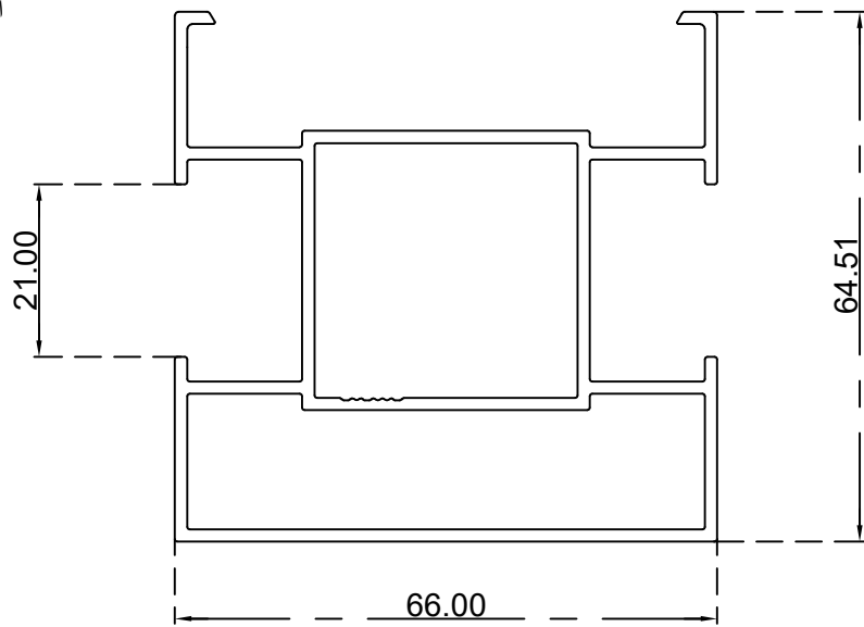
اطار باب مع غطاء الرقم التسلسلي للصنف: BLT3621 الوزن 1.401:(Kg/m)
