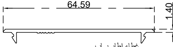
غطاء اطار باب الرقم التسلسلي للصنف: BLT1405 الوزن 0.278:(Kg/m)
