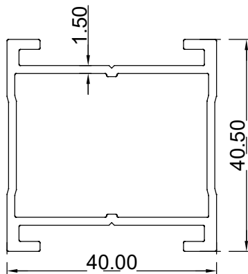
اطار باب بدون غطاء (40.5*40) ملم الرقم التسلسلي للصنف: BLT964 الوزن (Kg/m): 0.764
