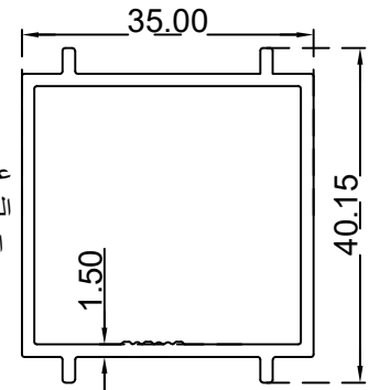
عمود تثبيت اطار باب الرقم التسلسلي للصنف: BLT3655 الوزن 0.593:(Kg/m)
