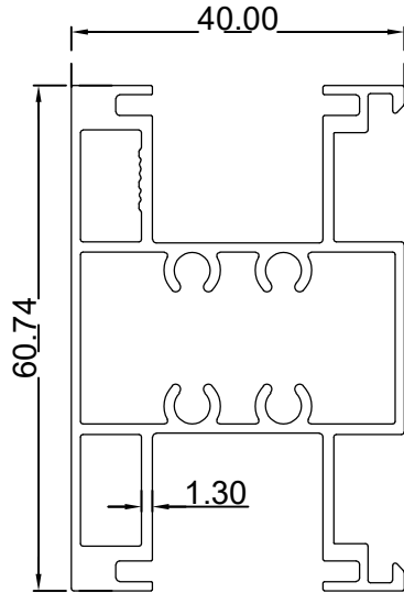
دفة و حلق جدار (40*60.74) ملم الرقم التسلسلي للصنف: BLT4282 الوزن 1.165:(Kg/m)
