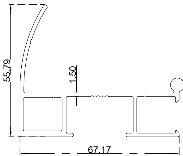
جدار ثمن ذكر مع غطاء الرقم التسلسلي للصنف: BLT3947 الوزن (Kg/m): 0.900
