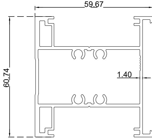
دفة و حلق جدار (60.74*59.67) ملم الرقم التسلسلي للصنف: BLT4301 الوزن 1.374:(Kg/m)
