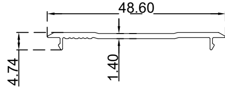
غطاء حلق جدار 48.59 ملم الرقم التسلسلي للصنف: BLT4280 الوزن 0.198:(Kg/m)
