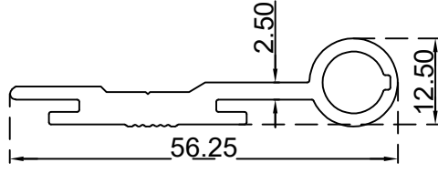
مفصلة دفة و حلق 40 ملم الرقم التسلسلي للصنف: BLT4619 الوزن 0.636:(Kg/m)
