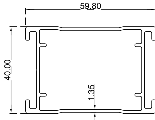
اطار باب بدون غطاء (40*59.8) ملم الرقم التسلسلي للصنف: BLT965 الوزن (Kg/m): 0.885
