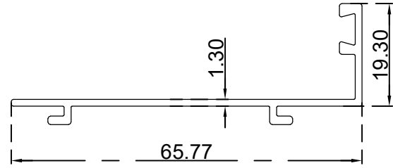
رداد باب 59.67 ملم الرقم التسلسلي للصنف: BLT4287 الوزن 0.380:(Kg/m)
