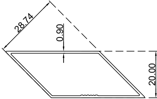
معين 20*30 ملم الرقم التسلسلي للصنف: BLT4843 الوزن 0.329:(Kg/m)
