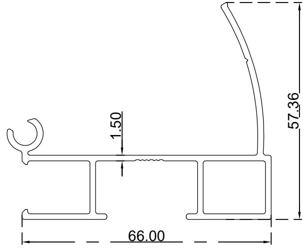
جدار ثمن انثى مع غطاء الرقم التسلسلي للصنف: BLT3948 الوزن (Kg/m): 0.895
