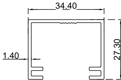
يو دربين (34.4*27.3) ملم الرقم التسلسلي للصنف: BLT4954 الوزن 0.421:(Kg/m)
