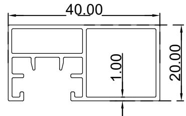
مستطيل كبس (20*40) ملم الرقم التسلسلي للصنف: BLT4336 الوزن 0.420:(Kg/m)
