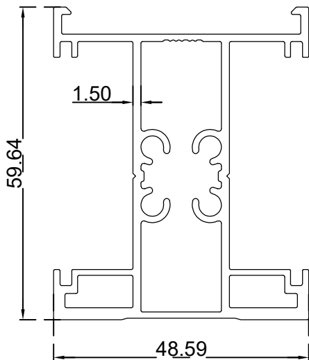
حلق جدار (48.59*59.64) ملم الرقم التسلسلي للصنف: BLT4283 الوزن 1.262:(Kg/m)
