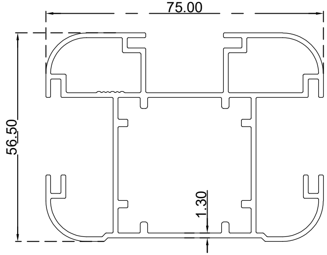
اطار باب ثلاثي (56.5*75) ملم الرقم التسلسلي للصنف: BLT4375 الوزن 1.514:(Kg/m)
