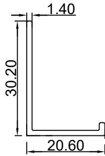
حلق باب كراج الرقم التسلسلي للصنف: BLT4448 الوزن 0.196:(Kg/m)
