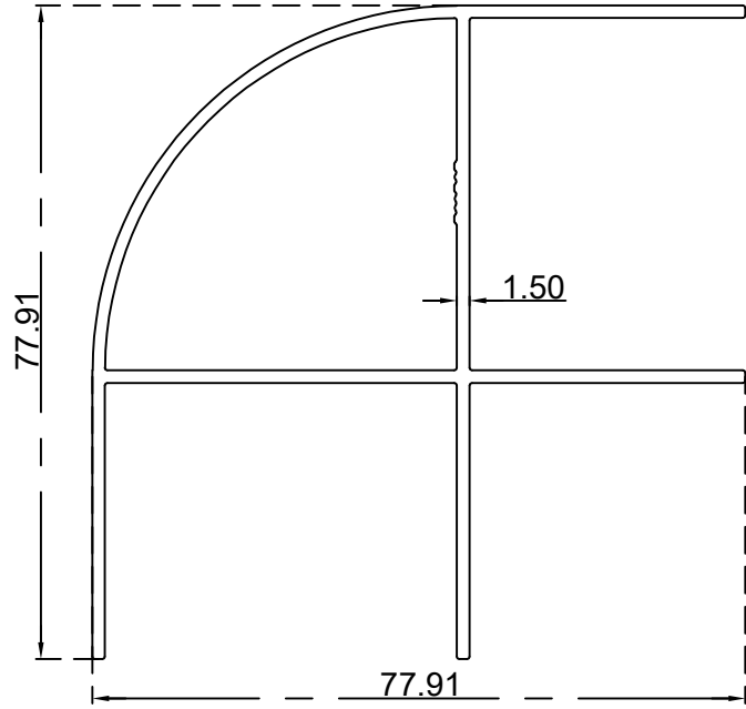
عمود زاوية ابواب خارجية الرقم التسلسلي للصنف: BLT4620 الوزن 1.176:(Kg/m)
