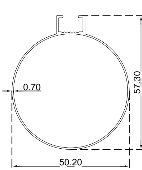
ديكور سقف دائري الرقم التسلسلي للصنف: BLT4794 الوزن 0.351:(Kg/m)
