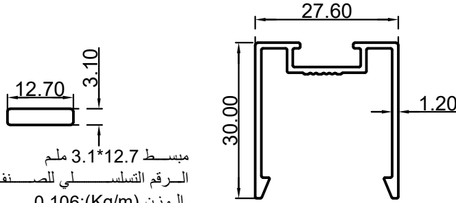
ديكور سقف 30 ملم الرقم التسلسلي للصنف: BLT4792 الوزن 0.330:(Kg/m)
