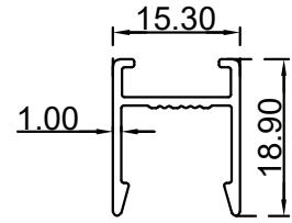
ديكور سقف 18.9 ملم الرقم التسلسلي للصنف: BLT4793 الوزن 0.162:(Kg/m)
