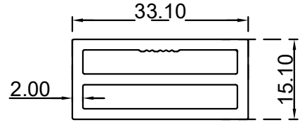
قاعدة ديكور داخلي الرقم التسلسلي للصنف: BLT4303 الوزن 0.643:(Kg/m)
