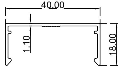
غطاء ديكور داخلي 40 ملم الرقم التسلسلي للصنف: BLT4304 الوزن 0.245:(Kg/m)
