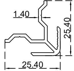
PL(25.4X25.4)mm الرقم التسلسلي للصنف: BLT4901 الوزن 0.269:(Kg/m)
