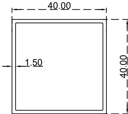
مربع (1.5*40*40) ملم الرقم التسلسلي للصنف: FG40X40X1.5 الوزن 0.629:(Kg/m)
