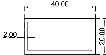
مستطيل (2*20*40) ملم الرقم التسلسلي للصنف: FG40X20X2C الوزن 0.609:(Kg/m)
