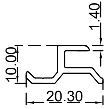
PL(20.3X10)mm الرقم التسلسلي للصنف: BLT4898 الوزن 0.145:(Kg/m)
