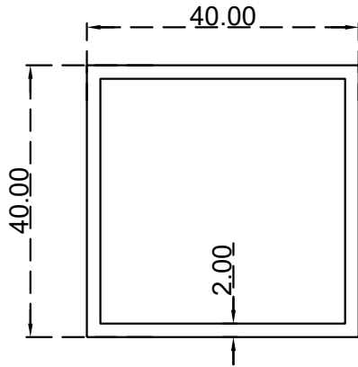
مربع 2*40*40 ملم الرقم التسلسلي للصنف: FG40X40X2B الوزن 0.824:(Kg/m)
