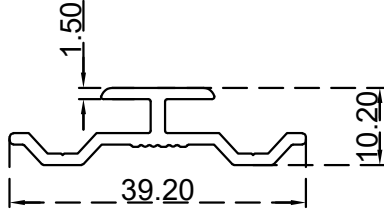
PL(39.2X10.2)mm الرقم التسلسلي للصنف: BLT4899 الوزن 0.265:(Kg/m)
