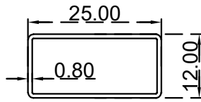
مستطيل (0.8*12*25) ملم الرقم التسلسلي للصنف: AS00083 الوزن 0.152:(Kg/m)
