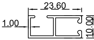
جسر برداية (10*23.6) ملم الرقم التسلسلي للصنف: BLT036 الوزن 0.177:(Kg/m)
