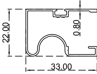
مقبض دفعة (22*33) ملم الرقم التسلسلي للصنف: BLT3376 الوزن 0.254:(Kg/m)
