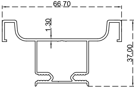
بروفيل طرفي (37*66.7) ملم الرقم التسلسلي للصنف: AS00090 الوزن 0.658:(Kg/m)
