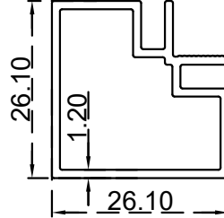
ربع مطبخ الرقم التسلسلي للصنف: BLT565 الوزن: 0.373:(Kg/m)
