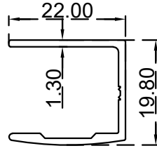
دفعة U الرقم التسلسلي للصنف: BLT3377 الوزن 0.223:(Kg/m)
