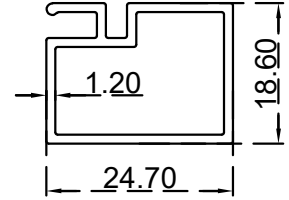
عمود زاوية الرقم التسلسلي للصنف: BLT1496 الوزن: 0.305:(Kg/m)
