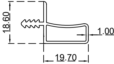
مقبض كيس (18.6*19.70) ملم الرقم التسلسلي للصنف: AS00080 الوزن 0.242:(Kg/m)
