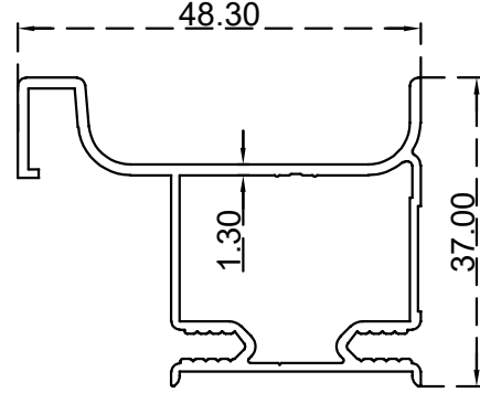
بروفيل طرفي (37*48.3) ملم الرقم التسلسلي للصنف: AS00089 الوزن 0.564:(Kg/m)
