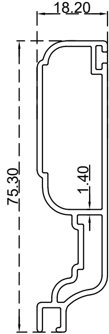
ثمان مطبخ الرقم التسلسلي للصنف: BLT091 الوزن: 0.426:(Kg/m)
