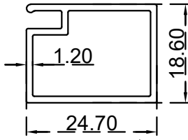
عمود جانبي الرقم التسلسلي للصنف: BLT1498 الوزن: 0.290:(Kg/m)
