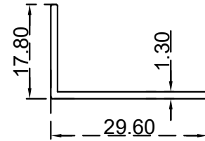
زاوية (1.3*17.8*29.6) ملم الرقم التسلسلي للصنف: AS00082 الوزن 0.163:(Kg/m)
