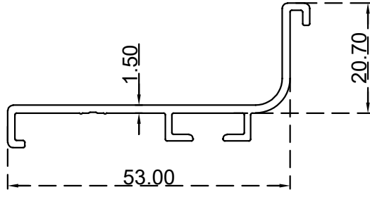
بروفيل طرفي (56.7*20.7) ملم الرقم التسلسلي للصنف: AS00078 الوزن 0.396:(Kg/m)
