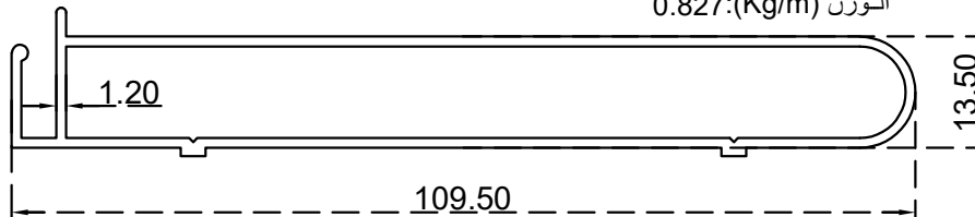
جرار مطبخ الرقم التسلسلي للصنف: BLT088 الوزن: 0.827:(Kg/m)
