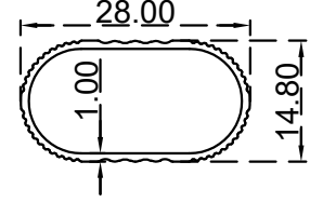
علاقة الرقم التسلسلي للصنف: BLT806 الوزن 0.164:(Kg/m)
