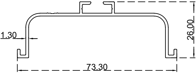
بروفيل طرفي (26*73.3) ملم الرقم التسلسلي للصنف: AS00077 الوزن 0.457:(Kg/m)
