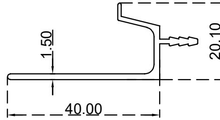
مقبض كيس L (40*20.1) ملم الرقم التسلسلي للصنف: AS00081 الوزن 0.304:(Kg/m)
