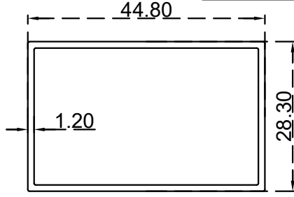
مستطيل (1.2*28.3*44.8) ملم الرقم التسلسلي للصنف: FG44.8X28.3X1.2 الوزن: 0.463:(Kg/m)
