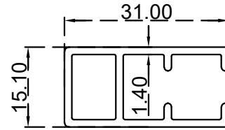
جسر برداية (15.1*31) ملم الرقم التسلسلي للصنف: BLT985 الوزن 0.374:(Kg/m)
