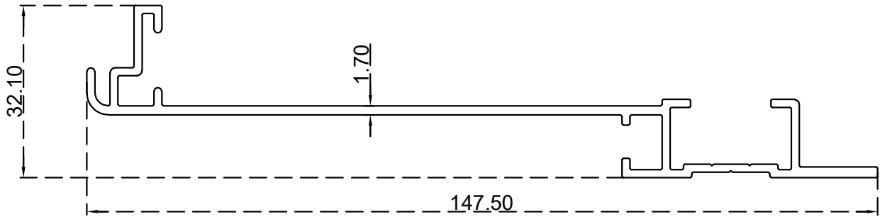
صندوق 100 ملم جومي الرقم التسلسلي للصنف: BLT867 الوزن 1.031:(Kg/m)
