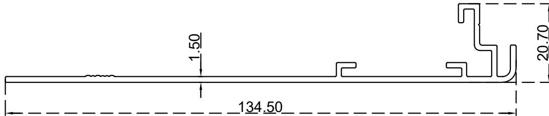
صندوق مسح جومي الرقم التسلسلي للصنف: BLT398 الوزن 0.756:(Kg/m)
