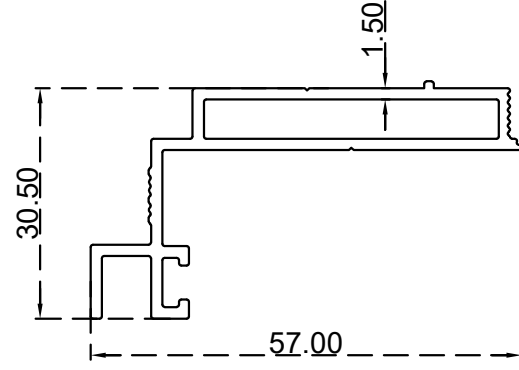
حلق صندوق أوبن آرت 30.5*47.5 ملم الرقم التسلسلي للصنف: BLT4983 الوزن (Kg/m): 0.610
