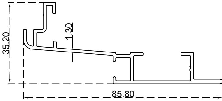
صندوق 40 ملم جومي الرقم التسلسلي للصنف: BLT1285 الوزن 0.624:(Kg/m)
