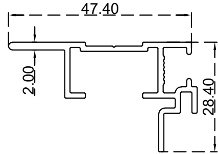
صندوق صفر جومي الرقم التسلسلي للصنف: BLT3233 الوزن 0.470:(Kg/m)
