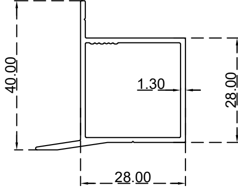
دفة صندوق أوبن آرت 40*40 ملم الرقم التسلسلي للصنف: BLT4991 الوزن (Kg/m): 0.473
