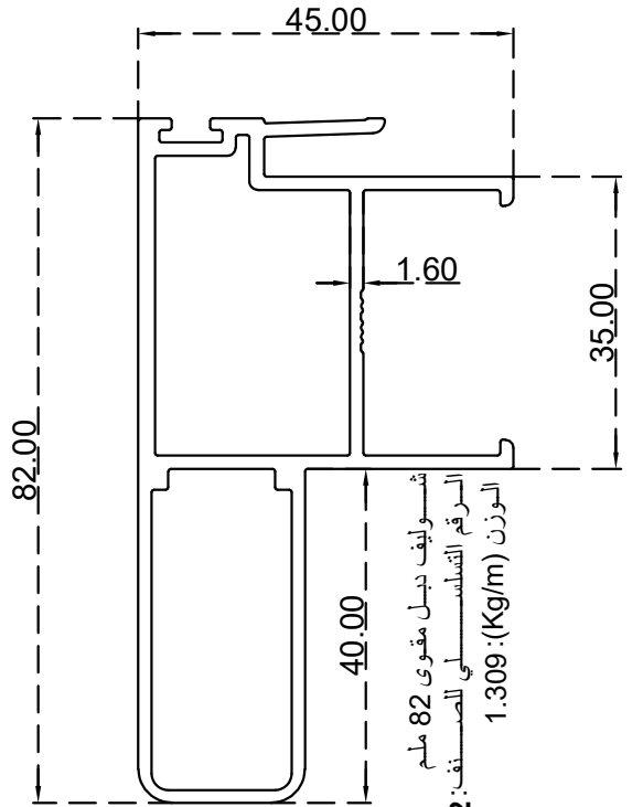
سادة مقوى عريض 75 ملم الرقم التسلسلي للصنف: BLT3507 الوزن 1.432:(Kg/m)
