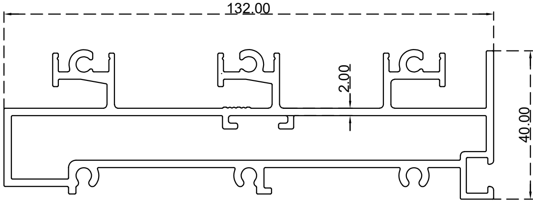
امباطية مفتوح ثلاث مجاري 40 ملم الرقم التسلسلي للصف: BLT4134 الوزن (Kg/m): 2.751
