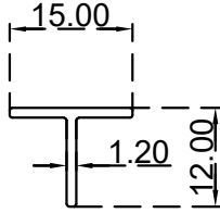
مقوي امباطية الرقم التسلسلي للصنف: T15X12X1.2 الوزن: 0.084 (Kg/m)
