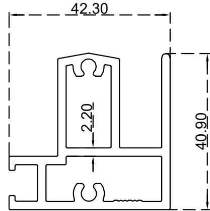
مجرى داخلي بانوراما 40 ملم الرقم التسلسلي للصنف: BLT3999 الوزن 1.257:(Kg/m)
