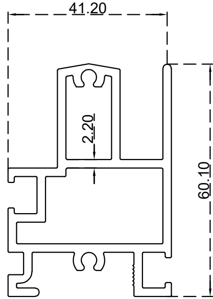
مجرى داخلي بانوراما 60 ملم الرقم التسلسلي للصنف: BLT562 الوزن 1.639:(Kg/m)
