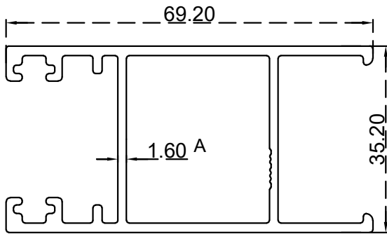
سادة دبل يد لف 24 ملم الرقم التسلسلي للصنف: BLT984A الوزن 1.126: (Kg/m)
