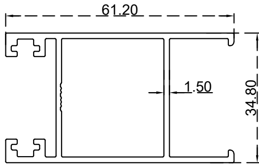
سادة دبل 24 ملم الرقم التسلسلي للصنف: ZD050A الوزن 0.908: (Kg/m)
