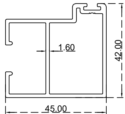
شوليف منخل الرقم التسلسلي للصنف: BLT3315 الوزن (Kg/m): 0.858
