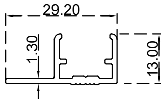
يو حلق الرقم التسلسلي للصنف: BLT3357 الوزن 0.217:(Kg/m)
