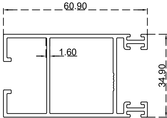
سادة مع فرشاية الرقم التسلسلي للصنف: BLT729 الوزن (Kg/m): 0.929
