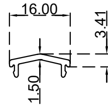
غطاء مجرى الرقم التسلسلي للصنف: BLT3930 الوزن 0.086:(Kg/m)
