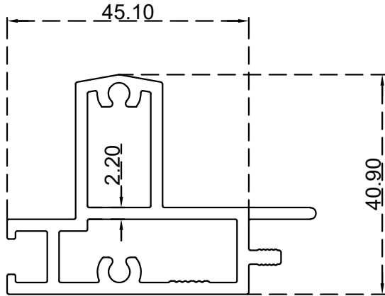
مجرى خارجي بانوراما 40 مل الرقم التسلسلي للصنف: BLT3998 الوزن 1.262:(Kg/m)
