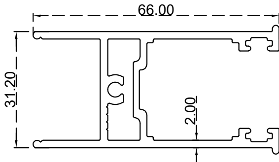
تحتون دبل بانوراما الرقم التسلسلي للصنف: BLT561 الوزن: 1.174 (Kg/m)
