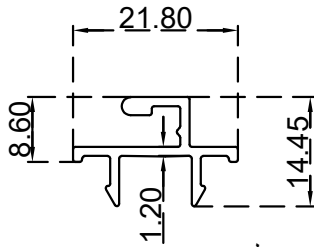
سن منخل الرقم التسلسلي للصنف: BLT033B الوزن (Kg/m): 0.184
