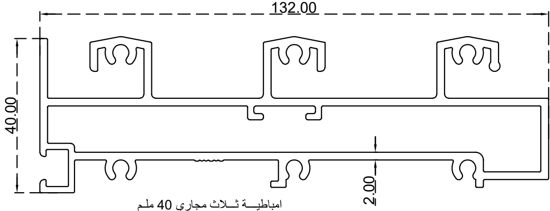
امباطية ثلاث مجاري 40 ملم الرقم التسلسلي للصف: BLT1575 الوزن (Kg/m): 2.749
