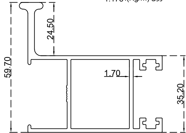
سادة دبل يد لف 59.7 ملم الرقم التسلسلي للصنف: BLT730 الوزن 1.2830: (Kg/m)
