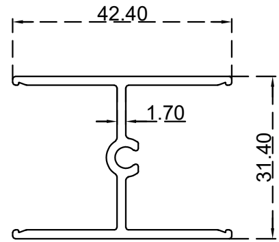
قاطع دبل 24 ملم الرقم التسلسلي للصنف: BLT725 الوزن (Kg/m): 0.619
