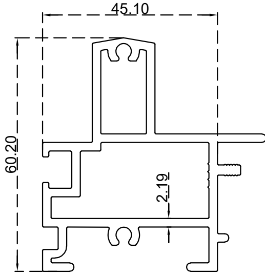
مجرى خارجي بانوراما 60 ملم الرقم التسلسلي للصنف: BLT563 الوزن 1.637:(Kg/m)
