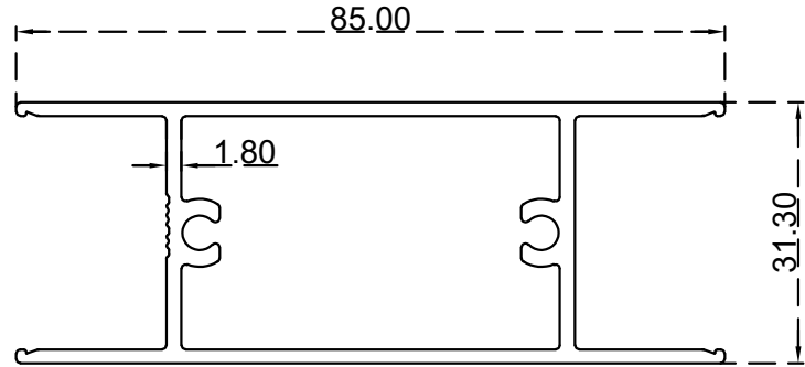
قاطع عريض دبل 85 ملم الرقم التسلسلي للصنف: BLT3623 الوزن (Kg/m): 1.143
