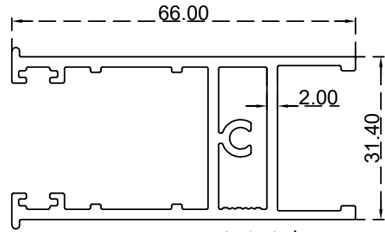
تحتون دبل بانوراما الرقم التسلسلي للصنف: BLT3743 الوزن 1.178: (Kg/m)
