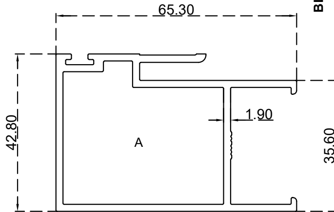
شوليف دبل ثقيل 24 ملم الرقم التسلسلي للصنف: BLT1599 الوزن 1.233:(Kg/m)
