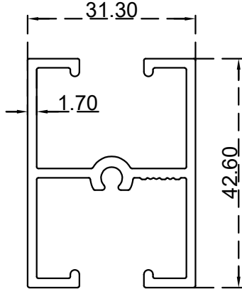
قاطع عادي (8-6) ملم الرقم التسلسلي للصنف: BLT727 الوزن: 0.742 (Kg/m)
