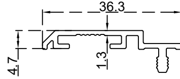
برواز الرقم التسلسلي للصنف: BLT3770 الوزن (Kg/m): 0.224
