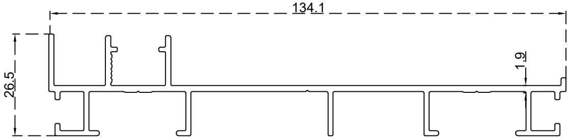
جنب ثلاث مجاري مفتوح الرقم التسلسلي للصنف: BLT3768 الوزن 1.080:(Kg/m)
