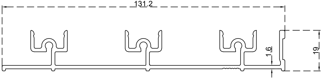
ارضية ثلاث مجاري 19 ملم الرقم التسلسلي للصنف: BLT3564 الوزن 1.290:(Kg/m)
