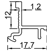
كليبس دفعة زجاج (11-7) ملم الرقم التسلسلي للصنف: BLT3567 الوزن 0.142:(Kg/m)
