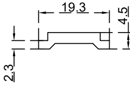
فلاخ الرقم التسلسلي للصنف: BLT1756 الوزن (Kg/m): 0.157
