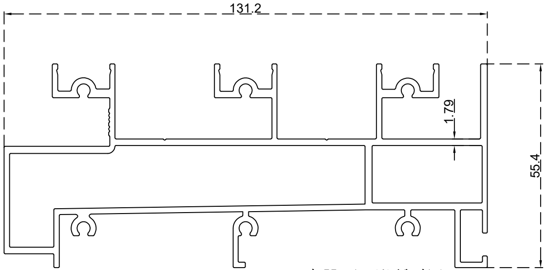
امباطية ثلاث مجاري 55 ملم الرقم التسلسلي للصنف: BLT3781 الوزن 2.645:(Kg/m)
