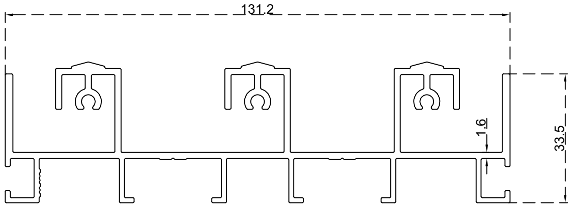
عليون ثلاث مجاري الرقم التسلسلي للصنف: BLT3771 الوزن 2.058:(Kg/m)
