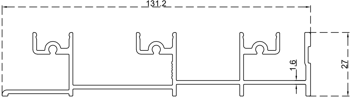
ارضية ثلاث مجاري 27 ملم الرقم التسلسلي للصنف: BLT1762 الوزن 1.445:(Kg/m)
