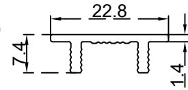
تي دبل الرقم التسلسلي للصنف: BLT031 الوزن (Kg/m): 0.158
