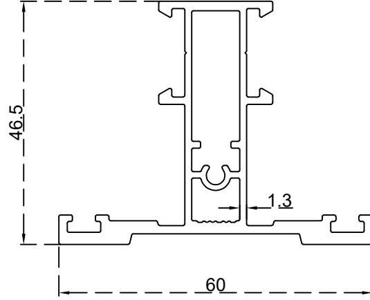
قاطع دفعة / دفعة الرقم التسلسلي للصنف: BLT761 الوزن (Kg/m): 0.990
