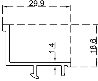
كليبس ثابت زجاج (6-3) ملم الرقم التسلسلي للصنف: BLT1979 الوزن 0.231:(Kg/m)
