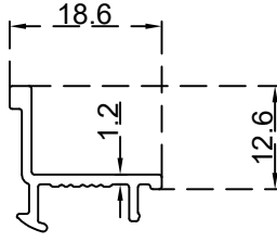
كليبس دفعة زجاج (4-6) ملم الرقم التسلسلي للصنف: BLT3218 الوزن (Kg/m): 0.145
