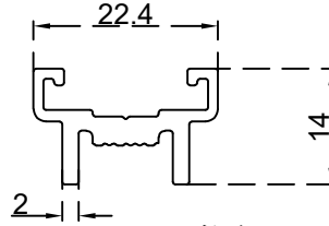
مجرى فلاح الرقم التسلسلي للصنف: BLT1770 الوزن 0.273:(Kg/m)
