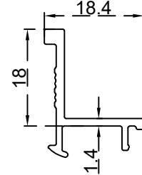
كليبس ثابت زجاج (18-13) ملم الرقم التسلسلي للصنف: BLT3163 الوزن 0.190:(Kg/m)
