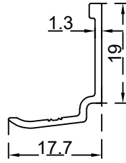
كليبس ثابت 2.4 ملم الرقم التسلسلي للصنف: BLT3419 الوزن 0.141:(Kg/m)
