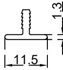
تي تسكيرة الرقم التسلسلي للصنف: BLT3660 الوزن (Kg/m): 0.086
