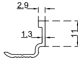
كليبس دفعة زجاج (33-28) ملم الرقم التسلسلي للصنف: BLT3600 الوزن 0.115:(Kg/m)
