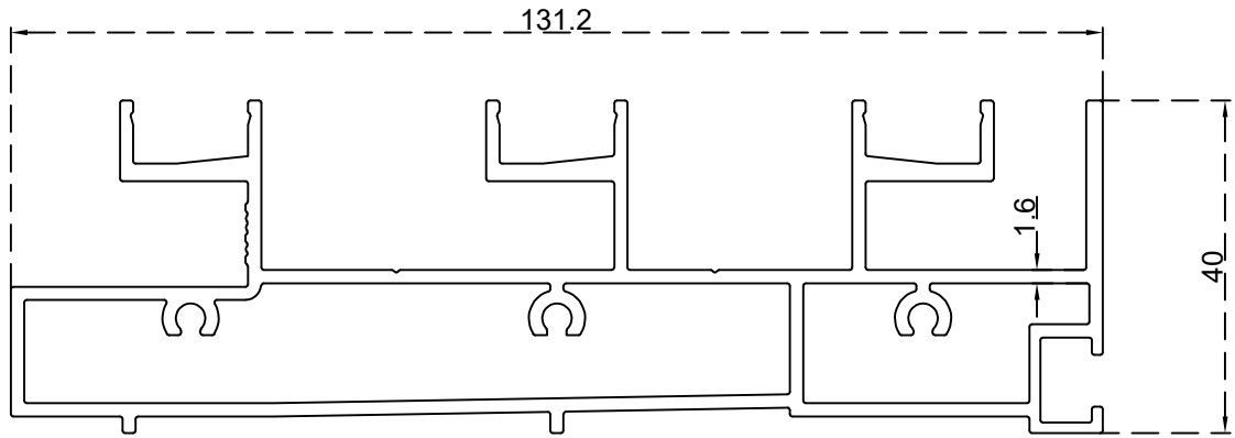
امباطية ثلاث مجاري 40 ملم الرقم التسلسلي للصنف: BLT3780 الوزن 2.320:(Kg/m)
