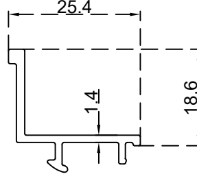
كليبس ثابت زجاج (11-6) ملم الرقم التسلسلي للصنف: BLT1901 الوزن 0.218:(Kg/m)
