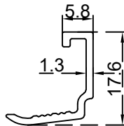
كليبس دفعة زجاج (18-14) ملم الرقم التسلسلي للصنف: BLT1767 الوزن 0.134:(Kg/m)
