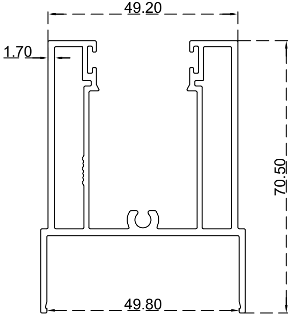
تحتون دبل (45-41) ملم الرقم التسلسلي للصنف: BLT3764 الوزن 1.422:(Kg/m)
