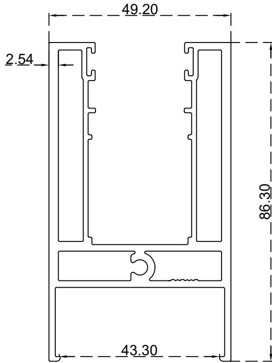
تحتون دبل مقوى (37-24) ملم الرقم التسلسلي للصف: BLT3757 الوزن 2.196:(Kg/m)
