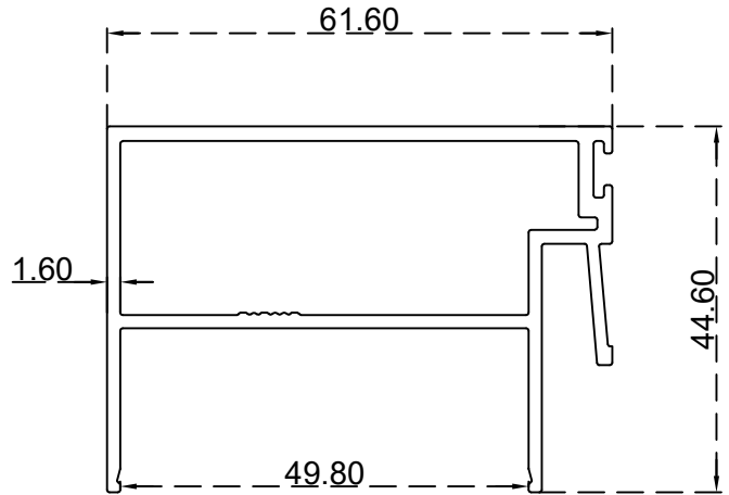
شوليف دبل (45-41) ملم الرقم التسلسلي للصنف: BLT3810 الوزن 1.025:(Kg/m)
