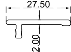
برواز مستقيم 27.5 ملم الرقم التسلسلي للصنف: BLT869 الوزن 0.190:(Kg/m)
