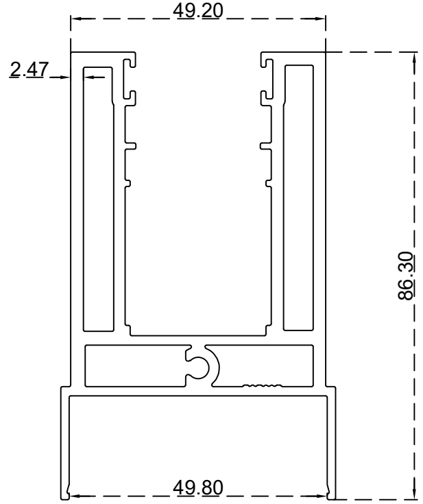
تحتون دبل مقوى (45-41) ملم الرقم التسلسلي للصنف: BLT3758 الوزن 2.464:(Kg/m)
