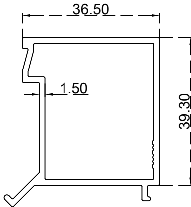
نوشيك اربع دفات الرقم التسلسلي للصف: BLT3760 الوزن 0.396:(Kg/m)
