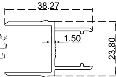
تحتون دبل (37-24) ملم الرقم التسلسلي للصف: BLT3801 الوزن 1.425:(Kg/m)
