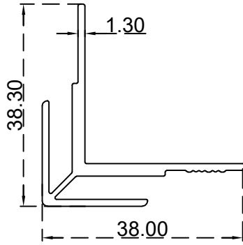
زاوية جمع الكيوند الرقم التسلسلي للصنف: BLT742 الوزن (Kg/m): 0.477
