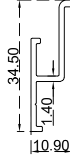
سقف مستعار (10.9*34.5) ملم الرقم التسلسلي للصنف: BLT616 الوزن (Kg/m): 0.215
