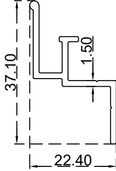
سقف مستعار (22.4*37.1) ملم الرقم التسلسلي للصنف: BLT615 الوزن (Kg/m): 0.286
