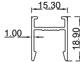
ديكور سقف 18.9 ملم الرقم التسلسلي للصنف: BLT4793 الوزن (Kg/m): 0.162
