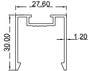
ديكور سقف 30 ملم الرقم التسلسلي للصنف: BLT4792 الوزن (Kg/m): 0.330
