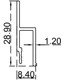
سقف مستعار (8.4*28.9) ملم الرقم التسلسلي للصنف: BLT503 الوزن (Kg/m): 0.167
