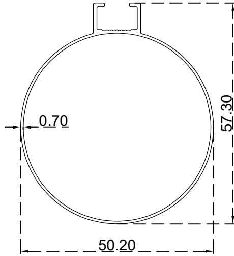
ديكور سقف دائري الرقم التسلسلي للصنف: BLT4794 الوزن (Kg/m): 0.351
