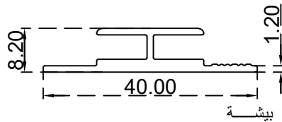
بيشة الرقم التسلسلي للصنف: BLT744 الوزن (Kg/m): 0.279
