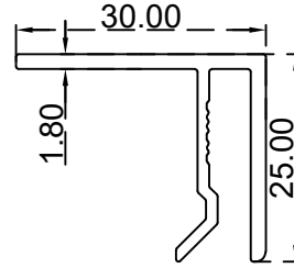
بروفيل تثبيت الكيوند الرقم التسلسلي للصنف: BLT3626 الوزن (Kg/m): 0.350
